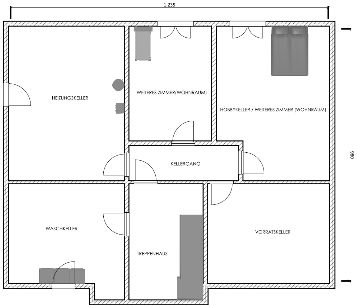
KELLERGESCHOSS
