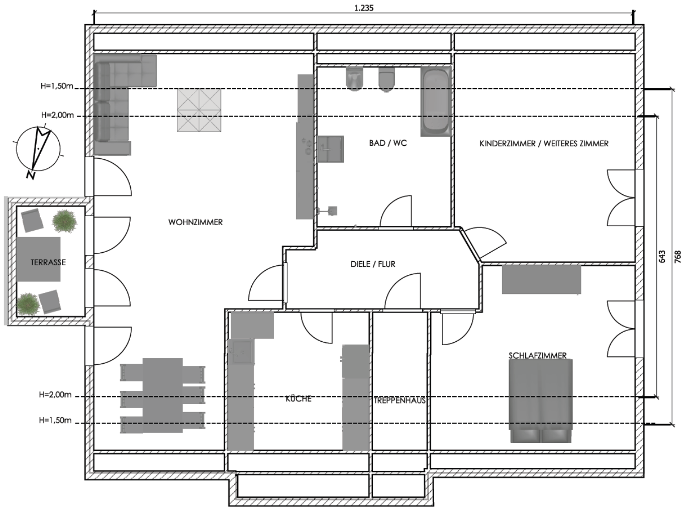
OBERGESCHOSS 103,5m 2
