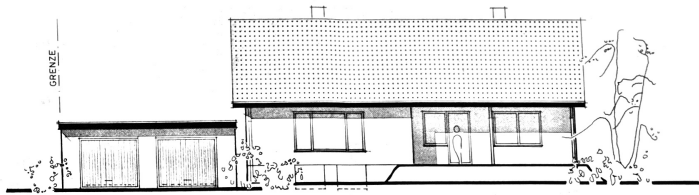
SÜDANSICHT
